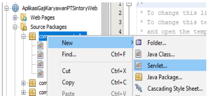
Gambar 278. Menambahkan Servlet
