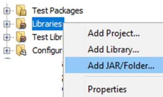
Gambar 276. Pilih Libraries
